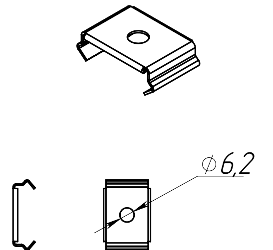
Скоба (только для IP40)
